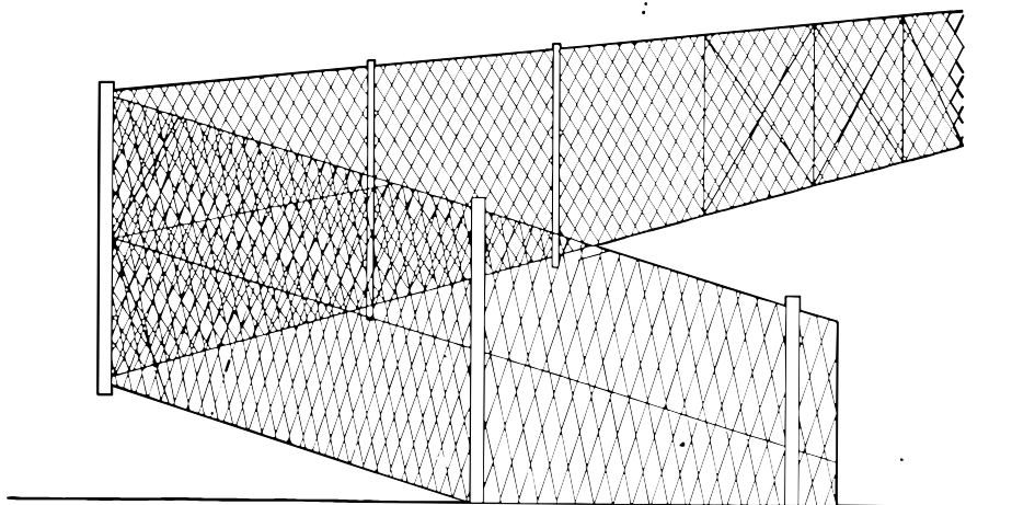
MEDIANERIAS LATERAL Y POSTERIOR
